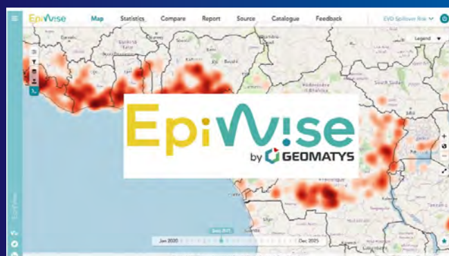
Plate-forme Epiwise pour les projections de risques épidémiques (Crédit: Geomatys)
